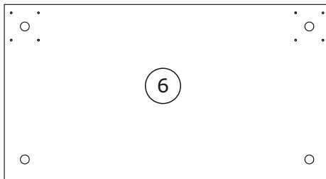
548x298x16 mm
